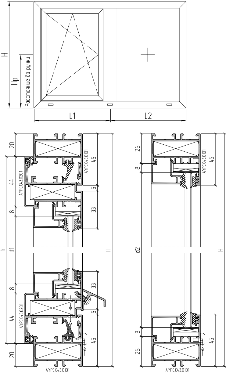
Пример расчета поворотно-откидного с боковой неоткрывающейся частью
