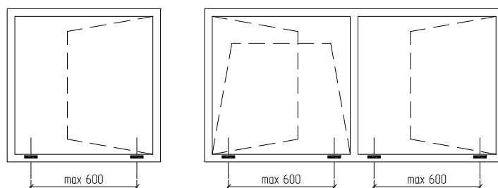
Схема расположения сливных отверстий
