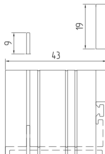
Обработка AUPC.C43.0202 и AUPC.C43.0203
