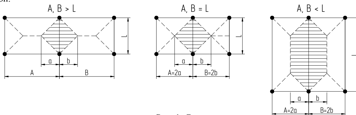
Рис. 1. Схемы нагрузок
