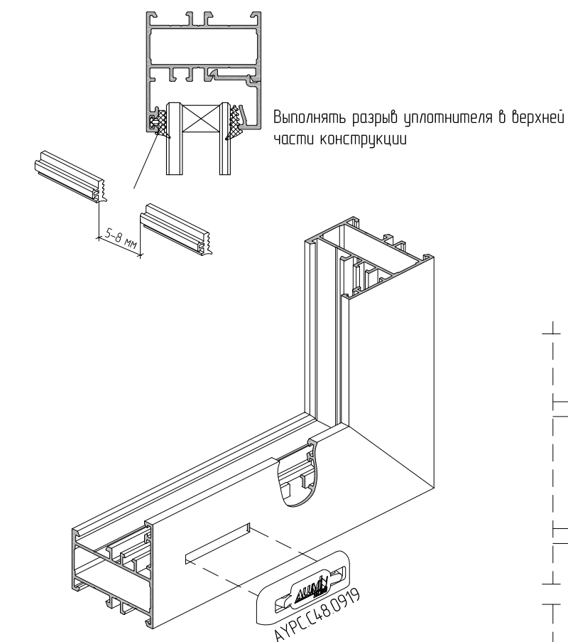
Схема расположения сливных отверстий
