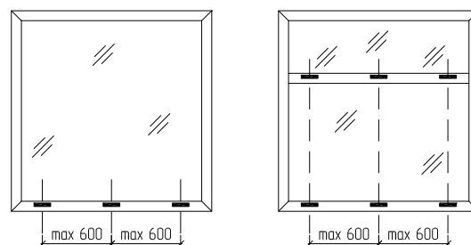
Схема расположения сливных отверстий
