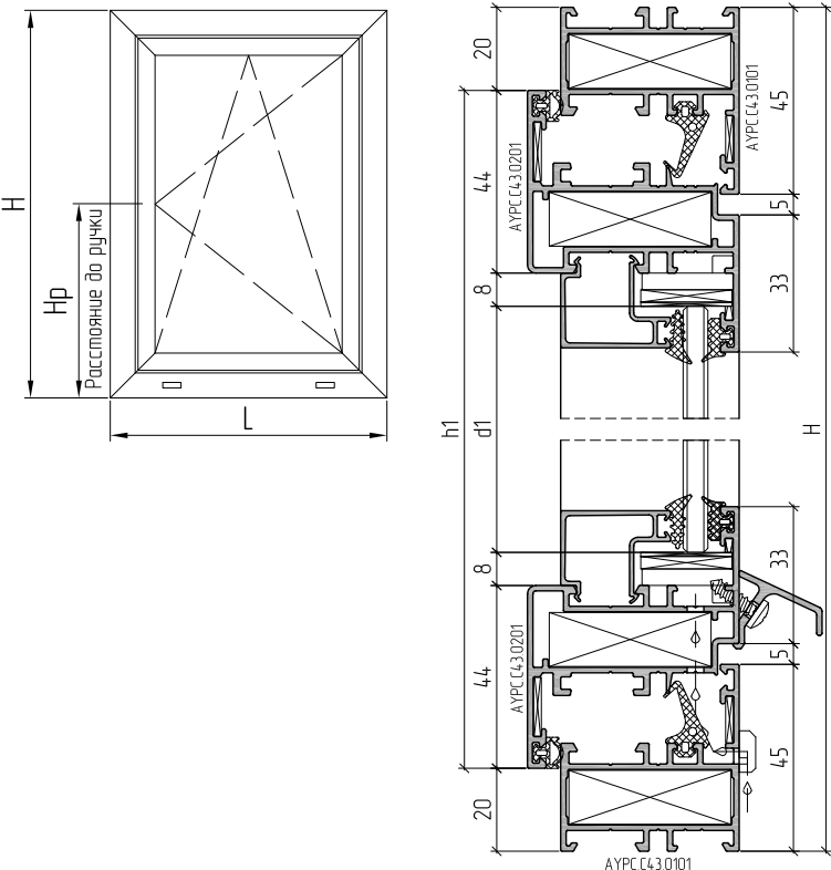
Пример расчета поворотно-откидного окна
