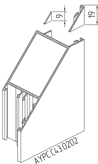
Обработка AUPC.C43.0202 и AUPC.C43.0203
