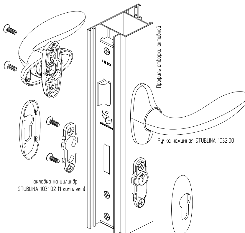
Установка ручки нажимной и накладки цилиндра
