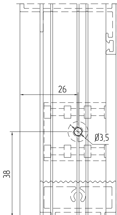
Дверь с порогом АУРС.С43.0805. Обработка рамы
